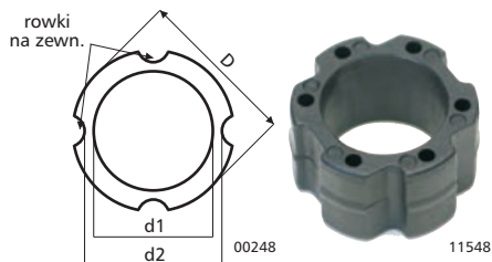
6E Okrągłe obrabiane zewnętrznie Round with external processing
