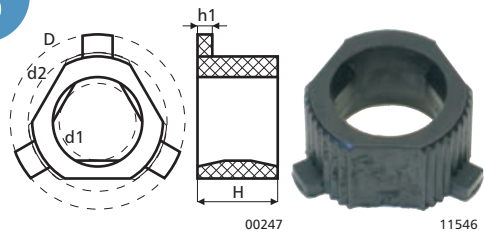
6A Trójkątne ze sprzężeniem Triangular with clutch
