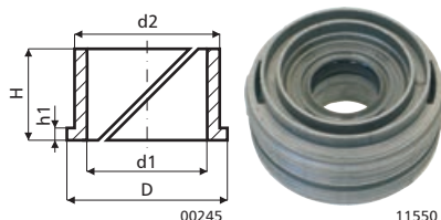
6D Okrągłe ze sprzężeniem Round with clutch
