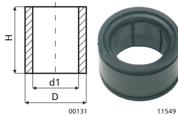
6B Okrągłe bez sprzężenka Round without clutch
